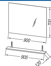
OG 90 / POL OG 90
