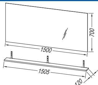
OG 150 / POL OG 150
