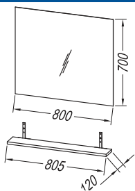
OG 80 / POL OG 80
