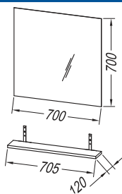
OG 70 / POL OG 70
