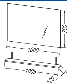
OG 100 / POL OG 100
